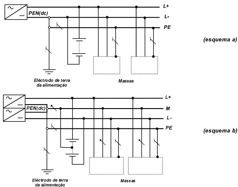
Fig. 31F — Esquema TN-S em corrente contínua (dc)
