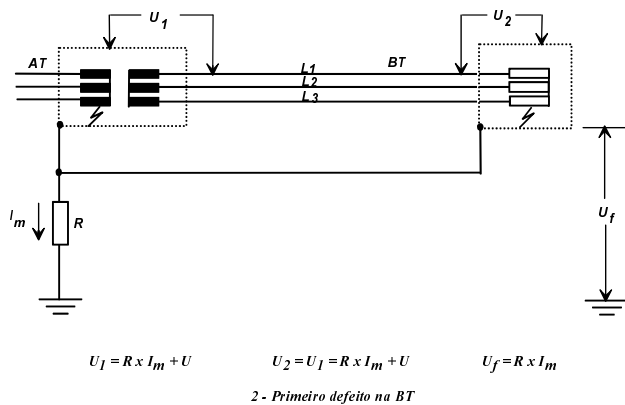
Figura 44K - Esquema IT, exemplo «e2»
