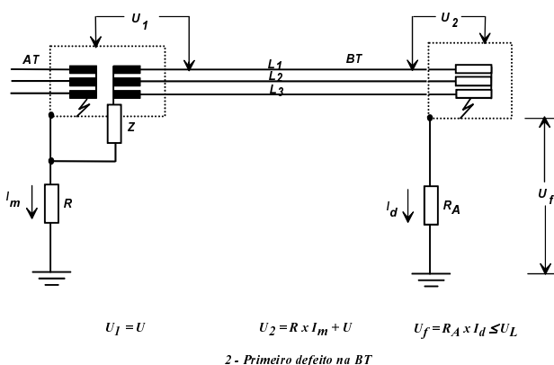
Fig. 44E — Esquema IT, exemplo «b»
