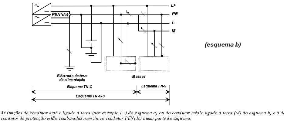
Fig. 31H — Esquema TN-C-S em corrente contínua (dc)
