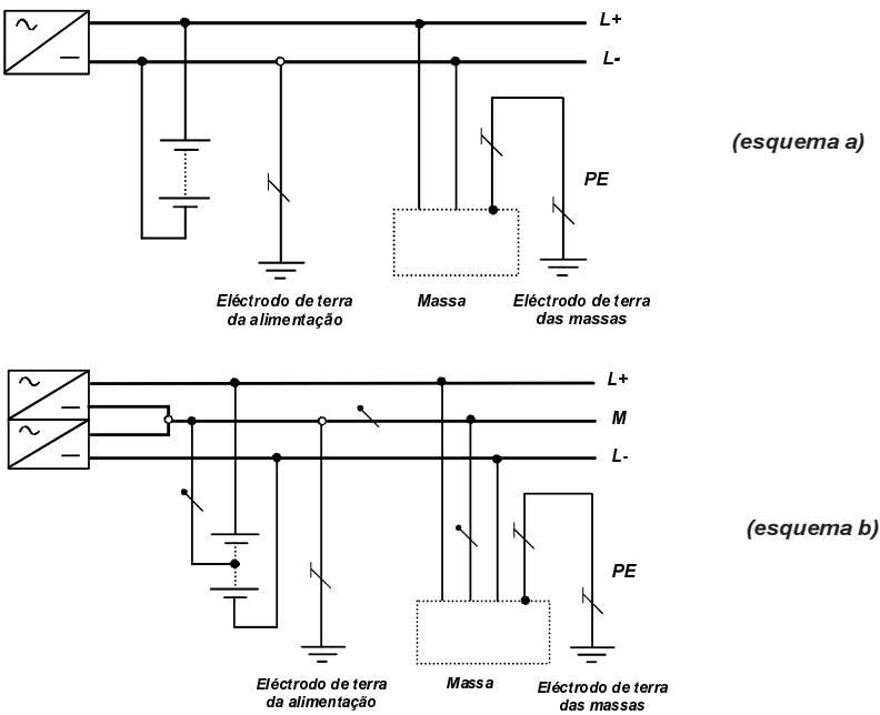
Figura 31 J — Esquema TT em corrente contínua (dc)
