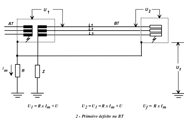
Figura 44J - Esquema IT, exemplo «e1»
