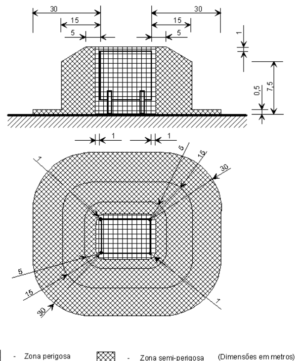
Fig. 801D — Zonas 1 (perigosa) e 2 (semi-perigosa) em reservatórios de gases sob pressão de densidade superior a 0,9, de altura superior a 7,5 m e de capacidade superior a 200 m 3 .
