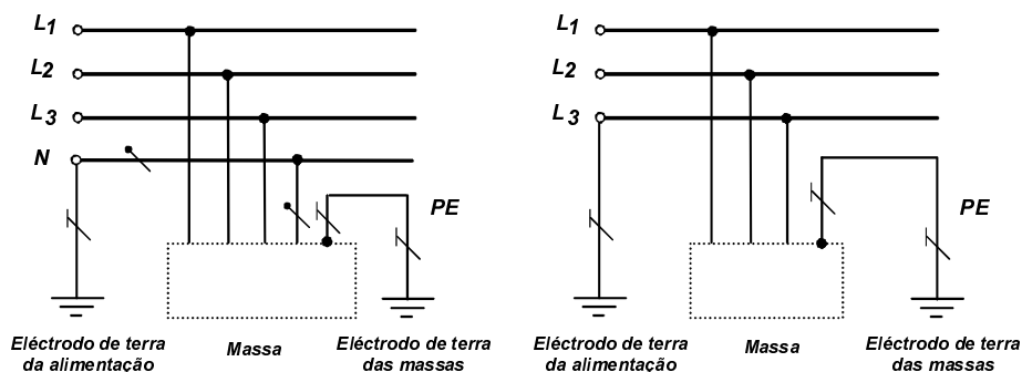
Fig. 31D — Esquema TT em corrente alternada (ac)
