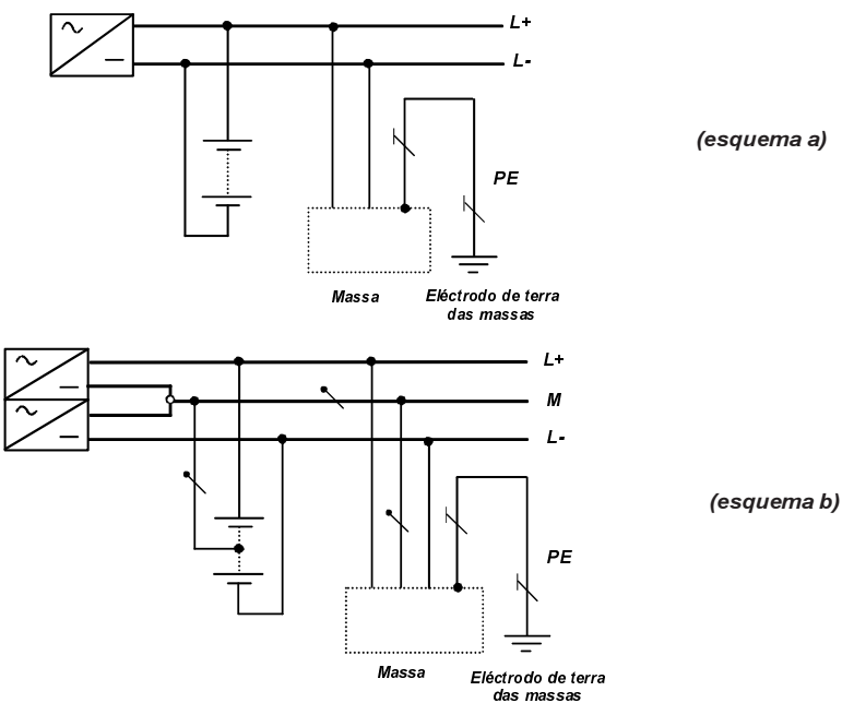
Figura 31 K — Esquema IT em corrente contínua (dc)
