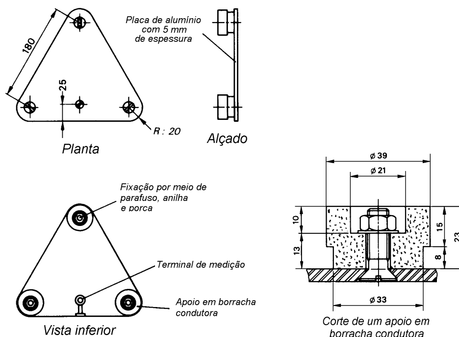
Fig. A1 — Eléctrodo de medição 2
