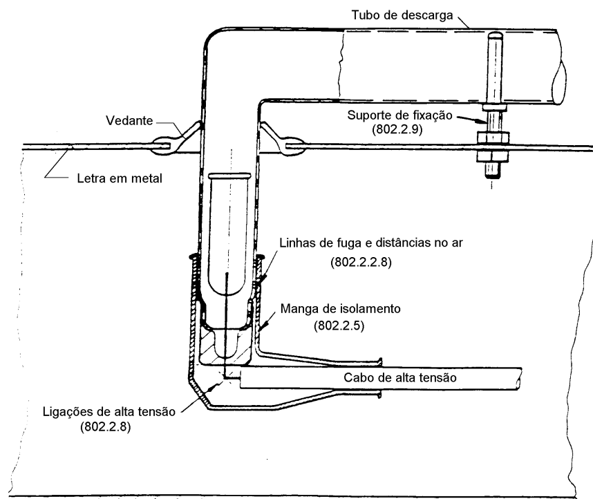
Fig. 3 — Exemplo de uma ligação de alta tensão com um electrodo a atravessar um painel metálico.
