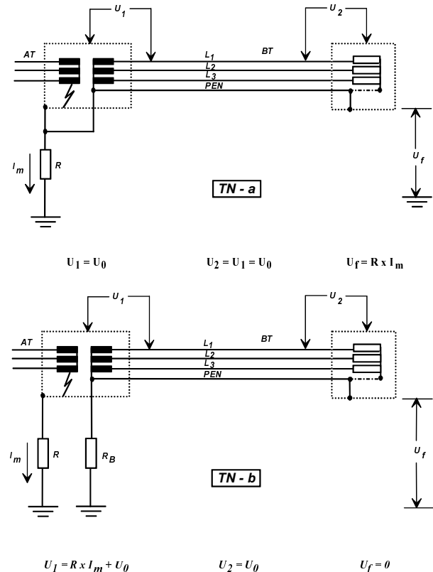
Fig. 44B — Esquema TN
