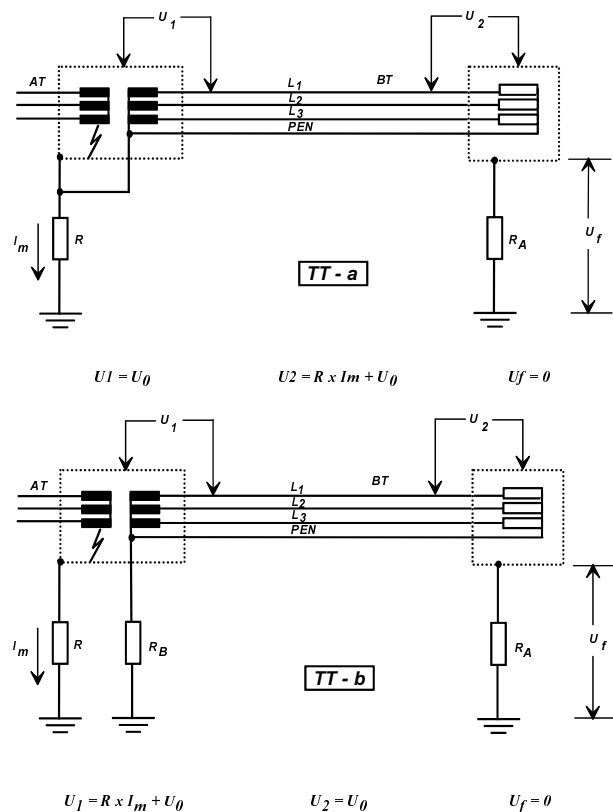
Fig. 44C — Esquema TT
