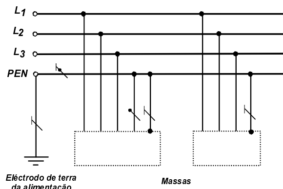
Fig. 31C — Esquema TN-C em corrente alternada (ac)
